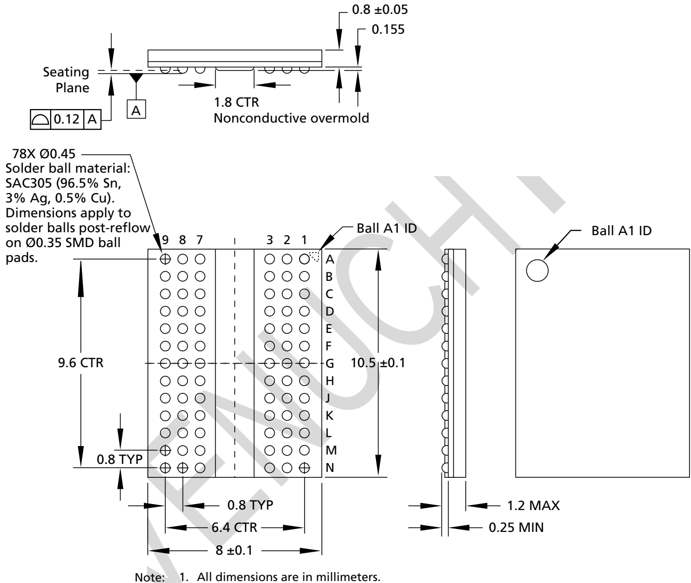
Figure 3: 78-Ball FBGA – x8; Die Rev. H, M, K (DA)
